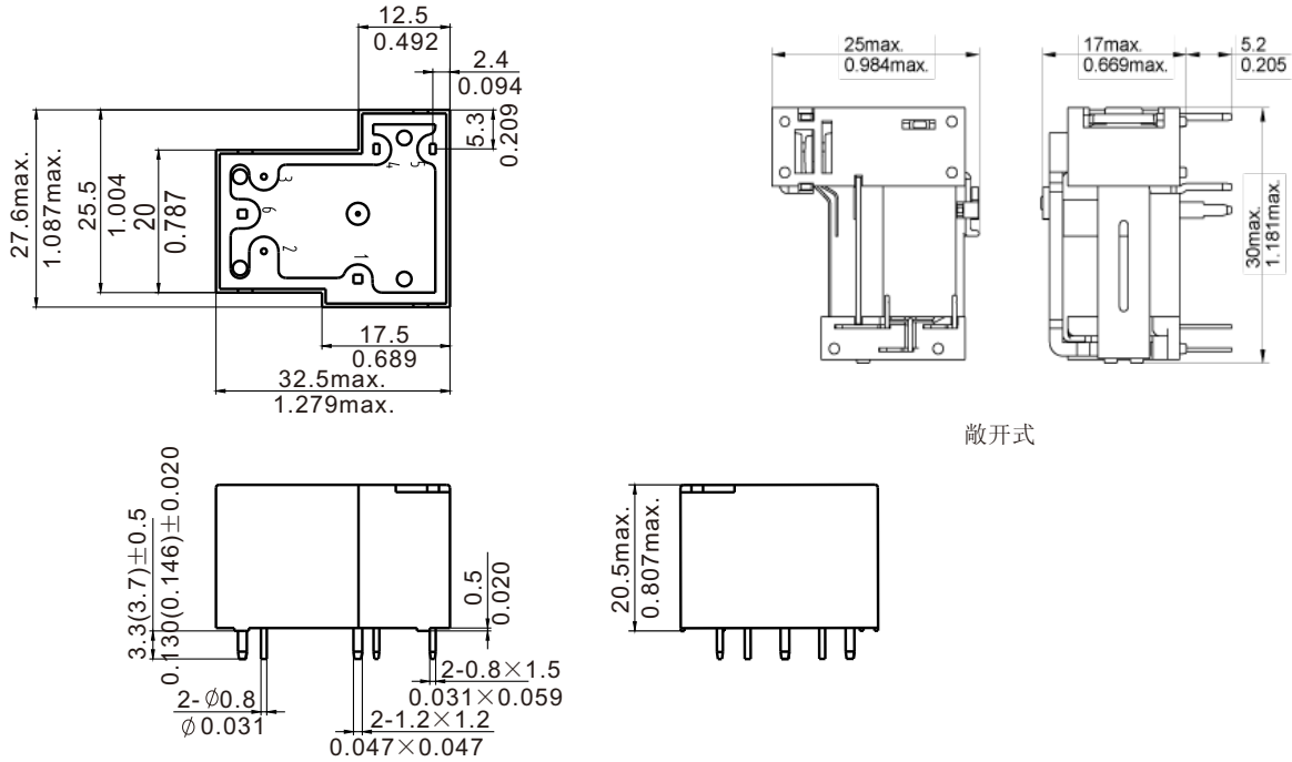
外形尺寸图
