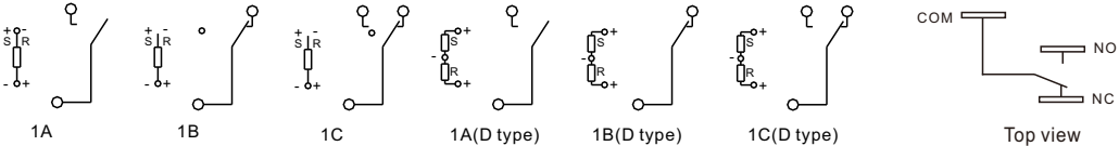
S:Set R:Reset
