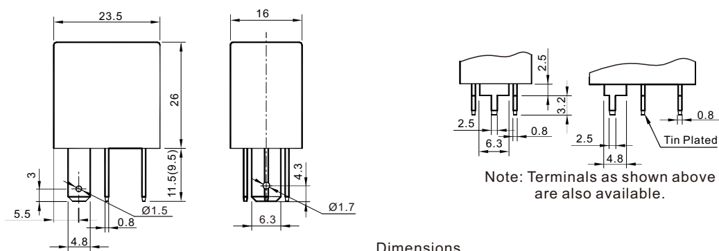
Dimensions
