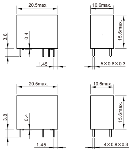
Dimensions
